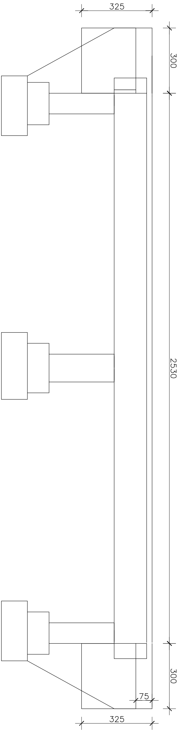
POPREČNI PRESJEK
