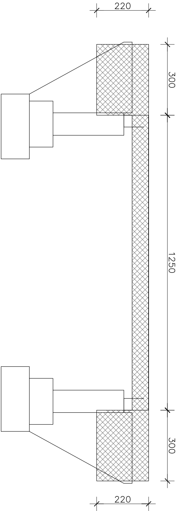
UZDUŽNI PRESJEK S BETONSKIM UTEGOM
