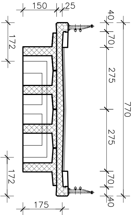
POPREČNI PRESJEK
