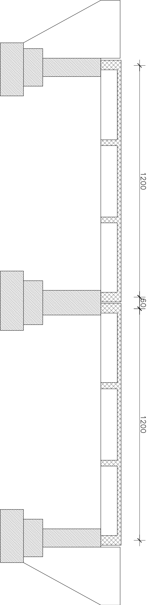
UZDUŽNI PRESJEK MOSTA 1
