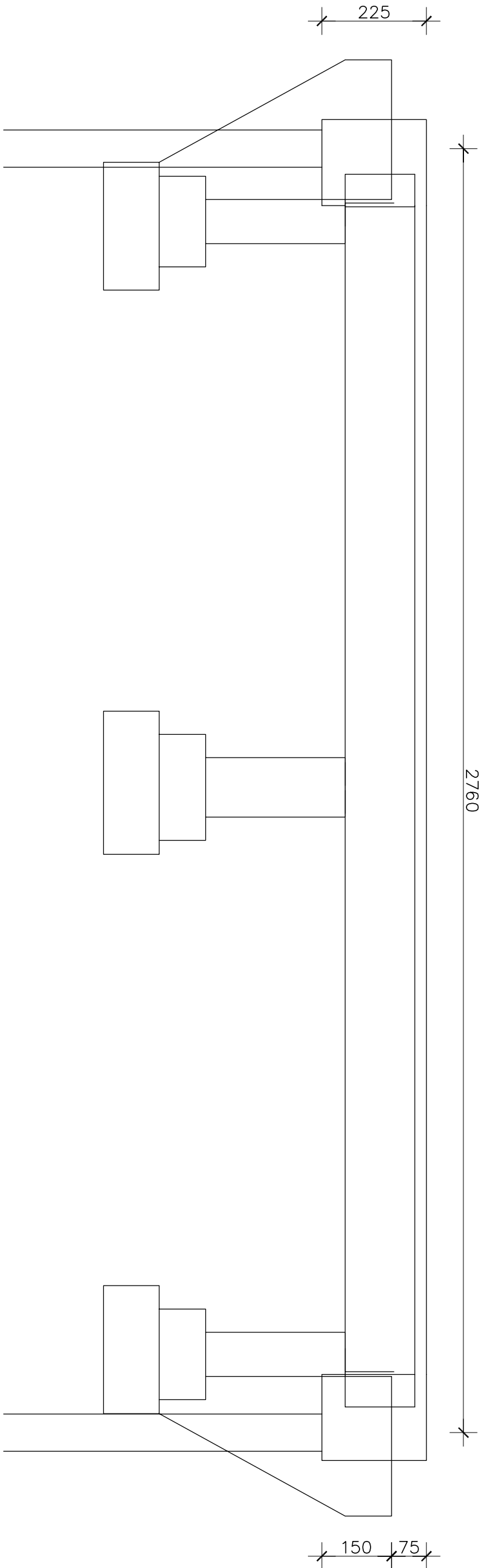
UZDUŽNI PRESJEK S PILOTIMA
